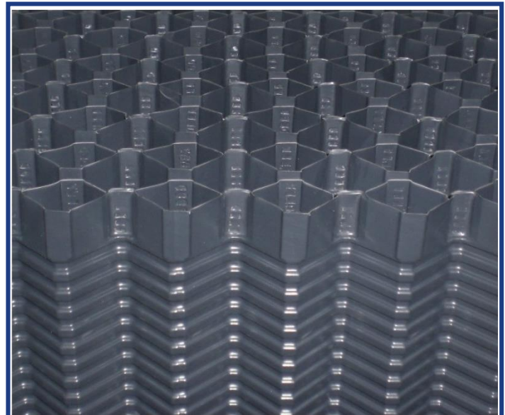
Senkrechte versetzte Kanäle 'offset flute'
